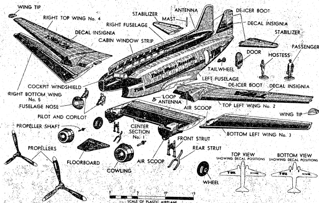
Kuva 1, josta jo osittain ilmenee kuinka äärettömän tarkkoja oikeitten koneitten jäljennöksiä nämä muoviset pienoismallit todella ovat.
