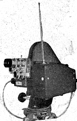
Kuva 2. Uusinta radio-ohjauksen alalta. Kauko-ohjattava Pathé-kaitafilmmikamera.
